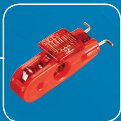
S2391 - Tiges métalliques vers l'extérieur : écartement de 11 à 13 mm
